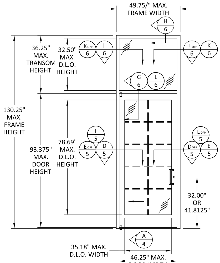
ELEVATION
