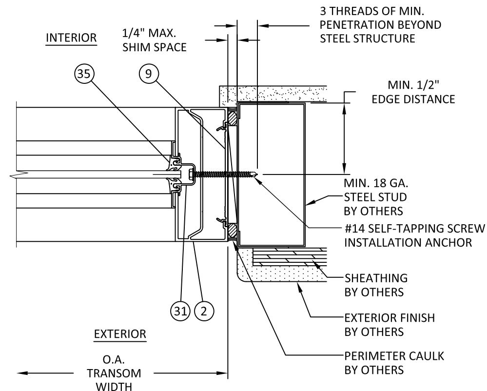
K 6 HORIZONTAL SECTION TRANSOM JAMB - STEEL STUD
