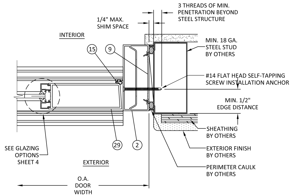
E 5 HORIZONTAL SECTION JAMB - STEEL STUD
