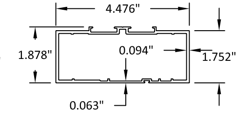
1A DOOR HEAD OHCC
