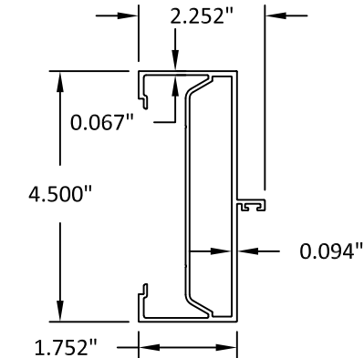
2 DOOR FRAME JAMB O/P
